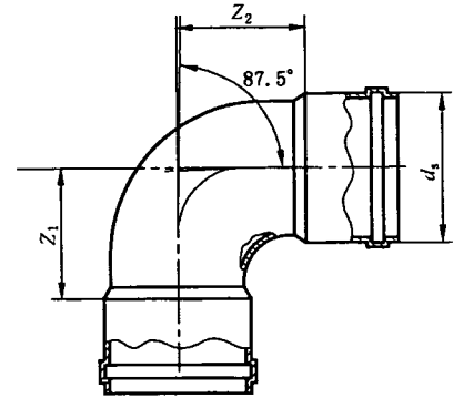
图 A.4 90^\circ 弯头
