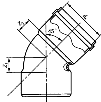
图 A.3 45^\circ 带插口弯头
