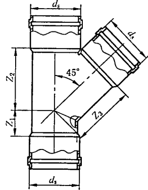
图 A.5 45°斜三通
