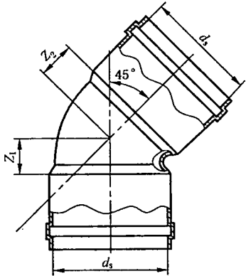
图 A.1 45^\circ 弯头
