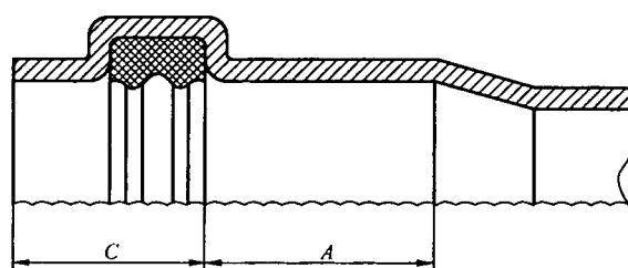
图 4 有效密封点的测量
