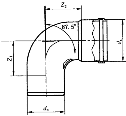
图 A.2 90^\circ 带插口弯头
