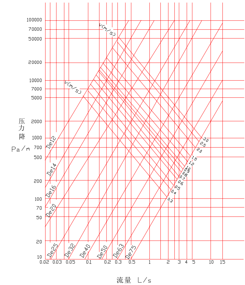
水温=65℃ 介质：水 图 A.0.3 热水管水力计算图表
