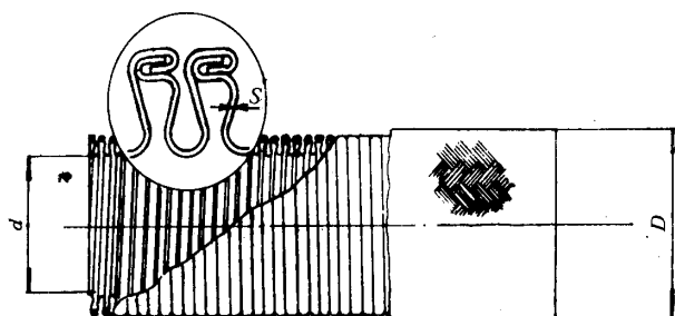
软管结构图
